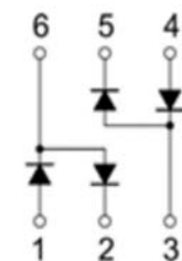
SOT-363
